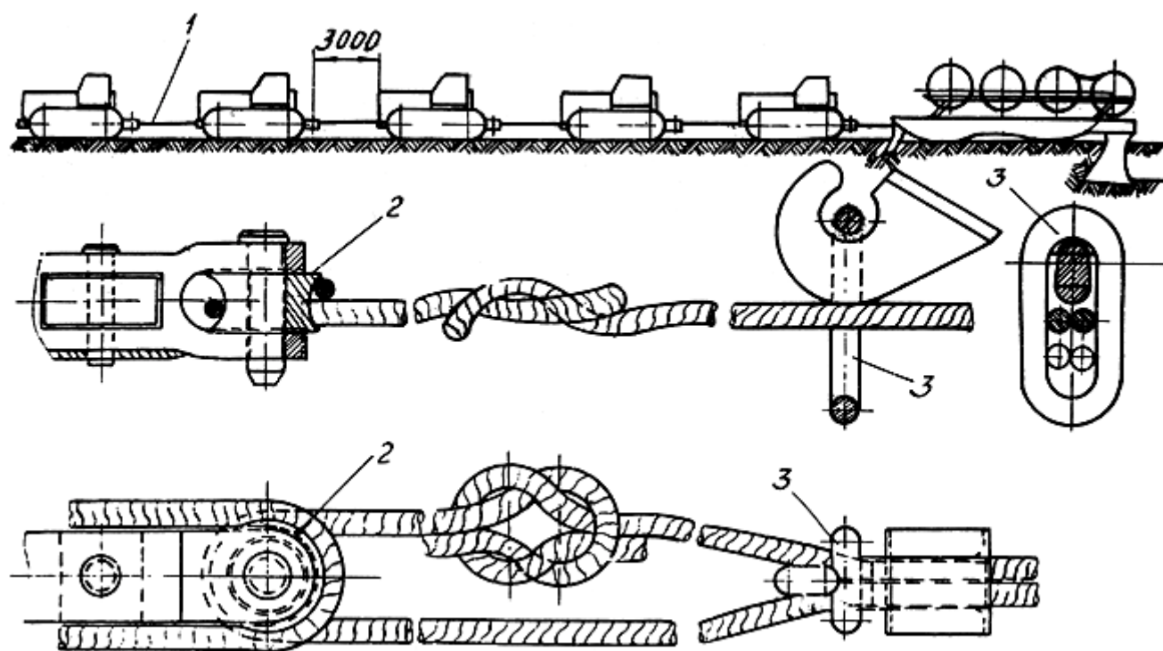
Рис. 2. Сцепка тракторов тросами:
