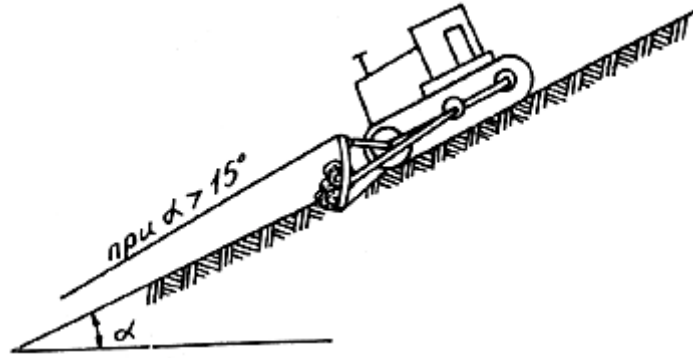
Рис.10. Схема использования бульдозера как якоря на уклоне
