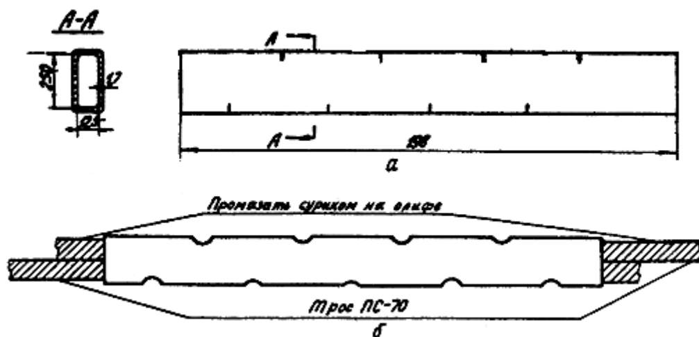
Рис.25. Сращивание троса ПС-70 с помощью овального соединителя:
