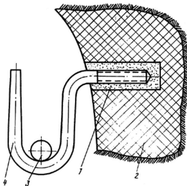
Рис. 14. Крепление крюков в тоннелях:
