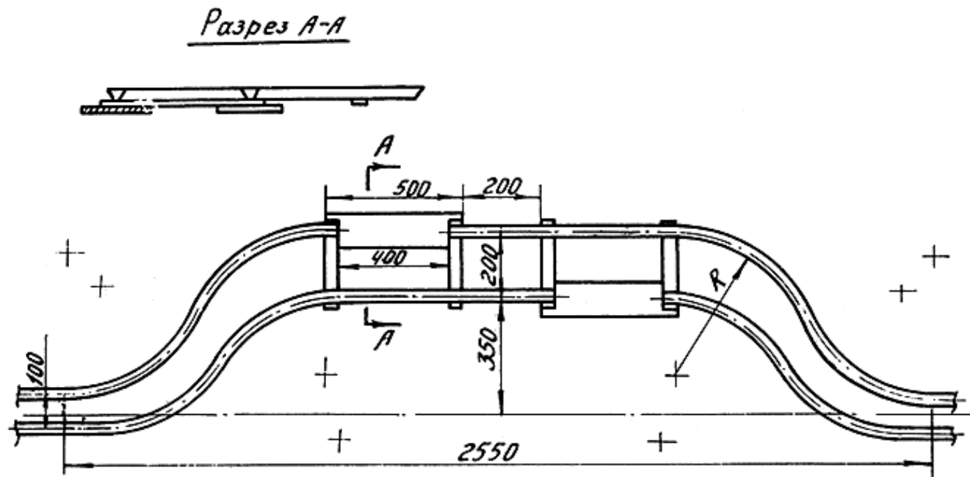
Рис. 23. Рама для закрепления выкладки кабеля
