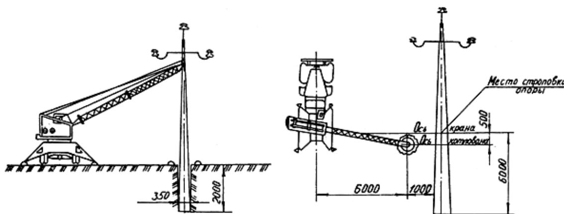
Рис. 28. Установка одностоечных опор ВЛ-6-10 кВ с помощью автомобильного крана
