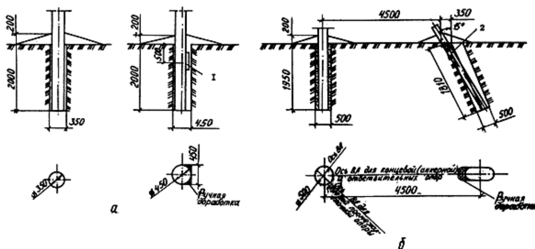
Рис. 27. Разработка котлованов:
