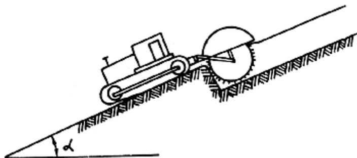
Рис.9. Схема работы на уклоне траншейного экскаватора
