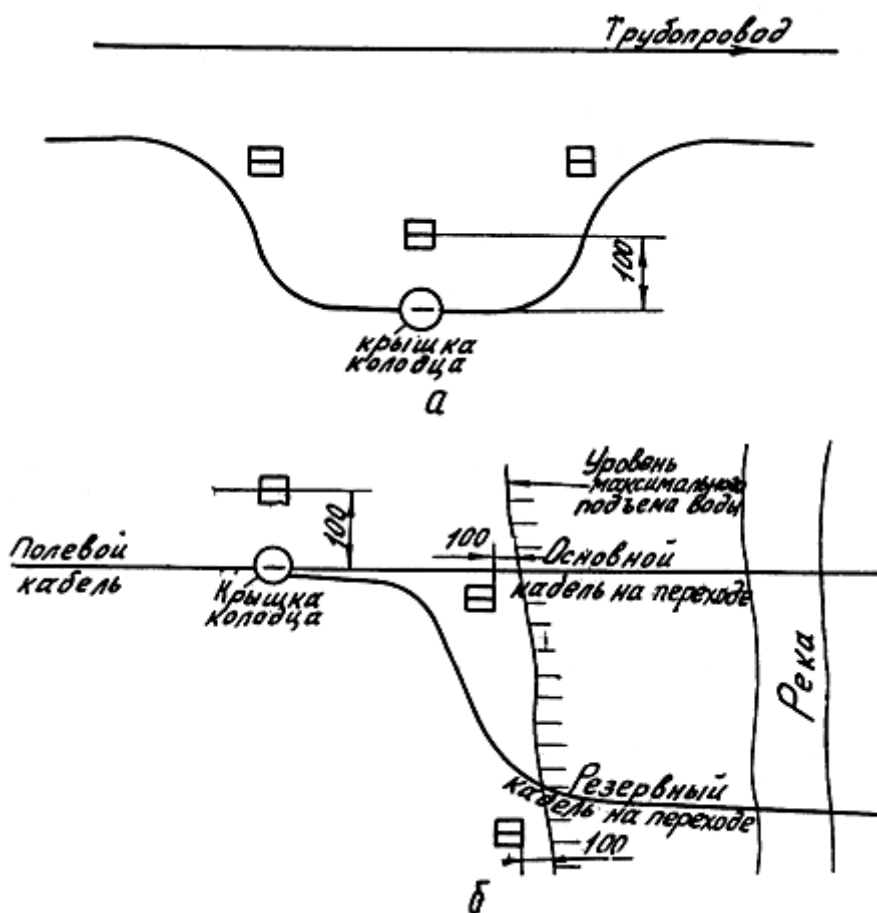
Рис. 17. Установка замерных столбиков у колодцев:
