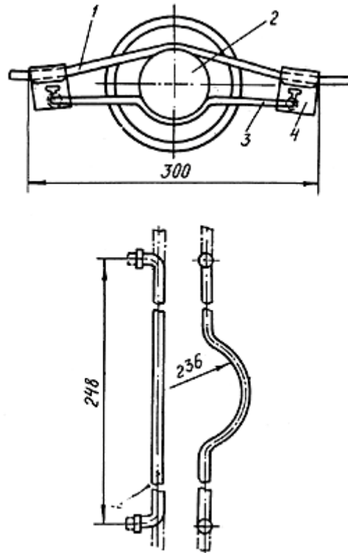
Рис. 33. Антивибрационный крюковой зажим ЗАК-10-1:
