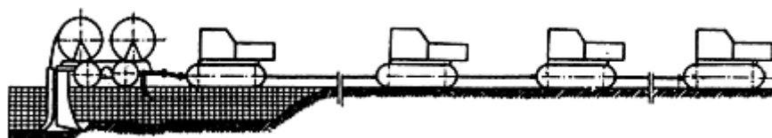
Рис.5. Обычная сцепка при работе на болотах I типа с твердого грунта
