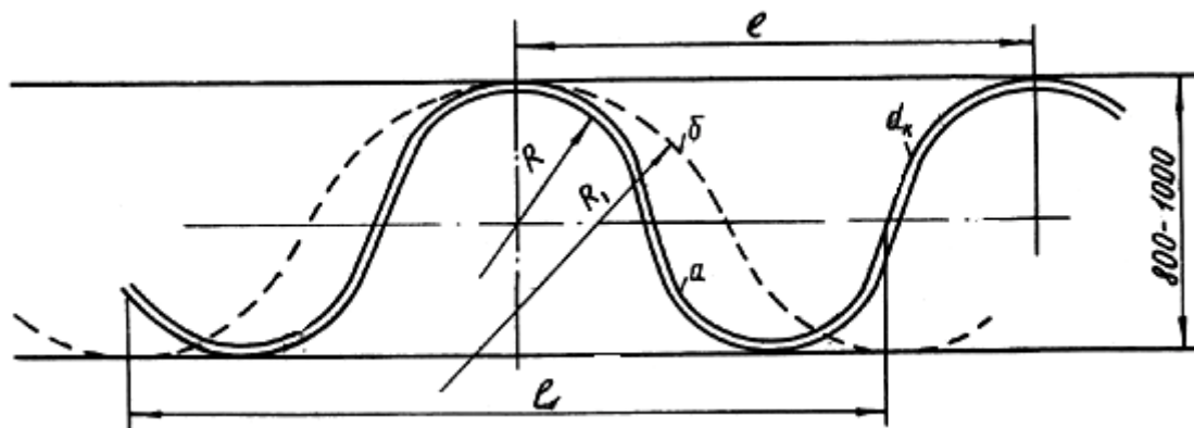
Рис.12. Прокладка кабеля в широкой траншее змейкой:
