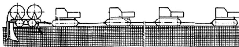
Рис 4. Разреженная сцепка при работе на болотах I типа
