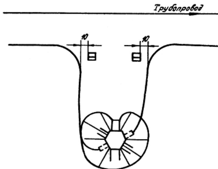
Рис. 21. Установка дополнительных столбиков у НУПа
