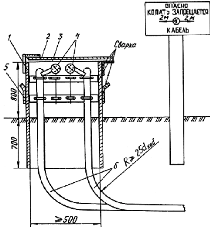
Рис.1. Оголовник для кабеля связи на подводных переходах (рекомендуемая конструкция):
