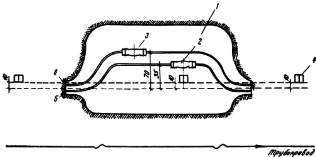
Рис. 16. Установка замерного столбика у муфт на двухкабельной линии связи:
