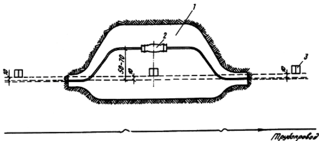
Рис. 15. Установка замерного столбика у муфты на однокабельной линии связи:
