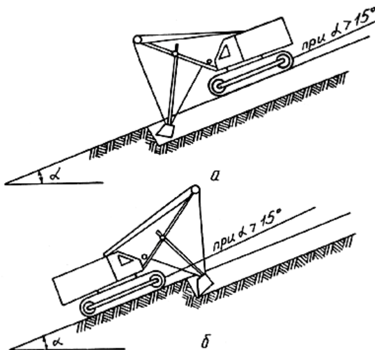
Рис.8. Схема работы на уклоне одноковшового экскаватора:
