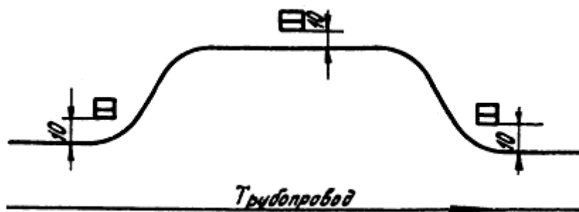
Рис. 19. Установка дополнительных столбиков на непродолжительных отклонениях трассы кабеля
