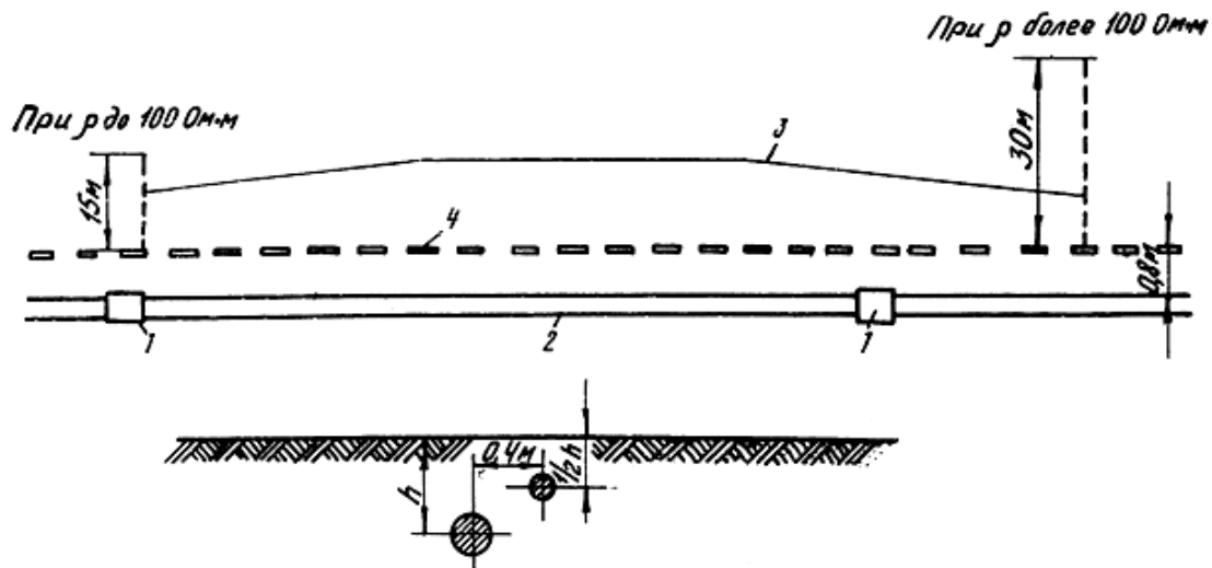
Рис. 24. Схема прокладки одного защитного провода (троса):
