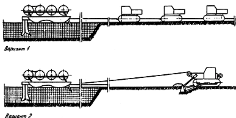
Рис.7. Обычная сцепка с длинным тросом при работе на болотах II-III типа
