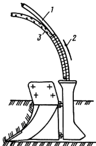
Рис.6. Связывание концов строительных длин кабеля:
