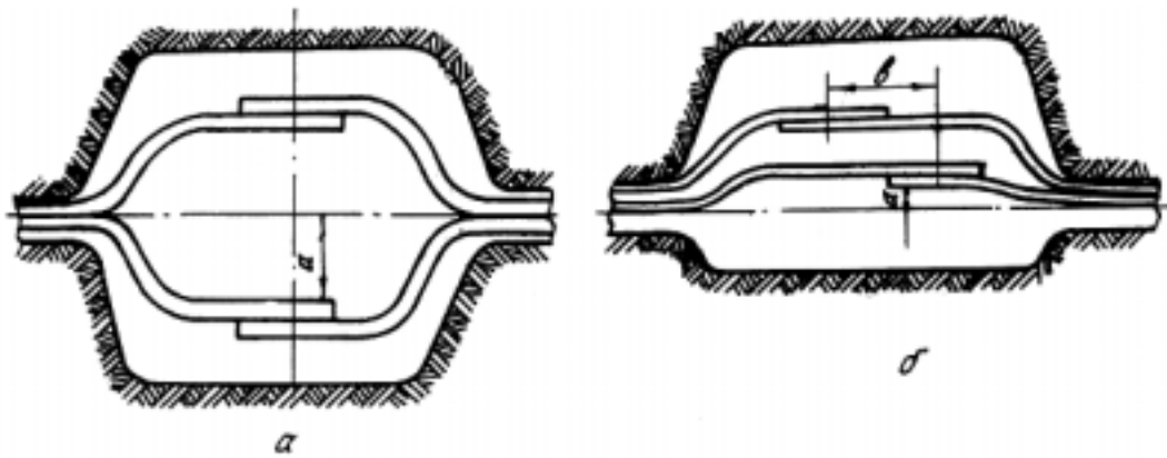
Рис. 22. Выкладка кабелей в котловане:
