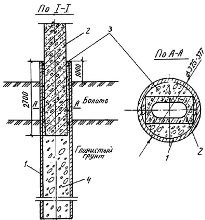
Рис. 29. Закрепление промежуточных опор на сваях:
