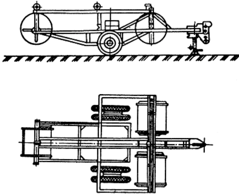
Рис.32. Одноосная трехбарабанная саморазгружающаяся раскаточная тележка грузоподъемностью 3 т; габариты: 4550х х2790х2100 мм
