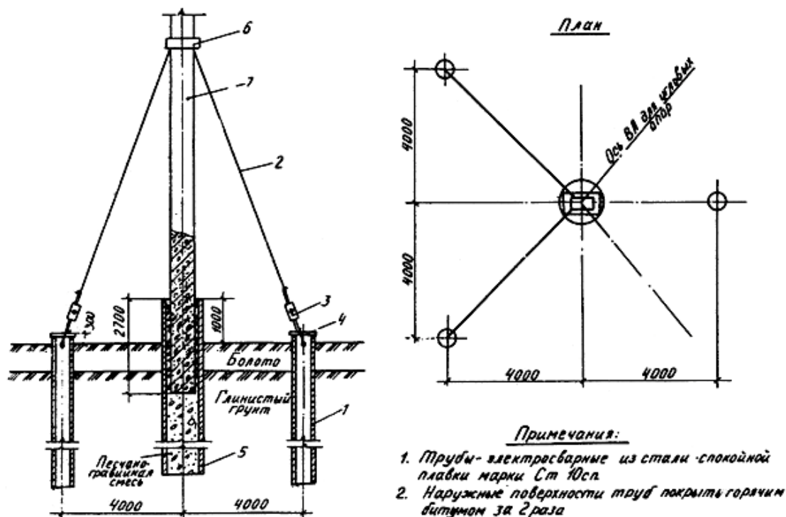
Рис. 30. Закрепление анкерно-угловых опор на болотах и пучинистых грунтах: 1 - труба диаметром 152 мм; 2 - оттяжка диаметром 16 мм; 3 - стяжной винт; 4 - заглушка; 5 - трубы диаметром 325-377 мм; 6 - хомут; 7 - железобетонная стойка
