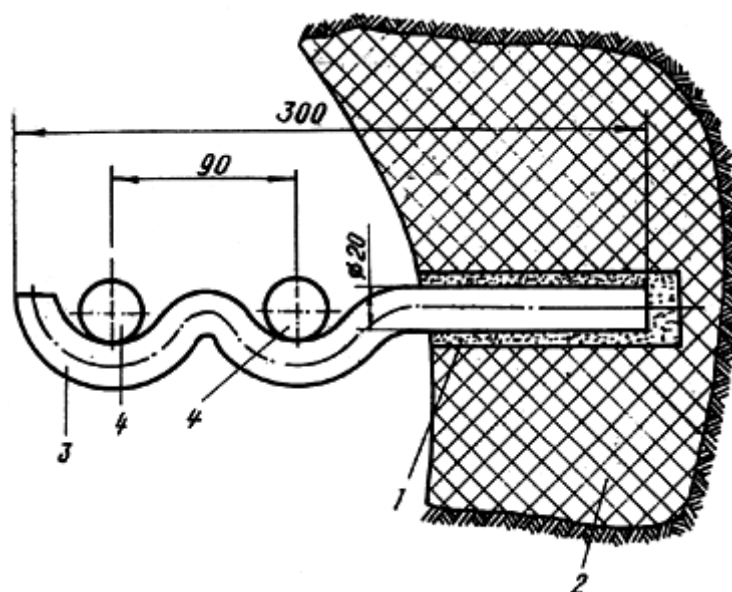
Рис.13. Крепление скоб в тоннелях:
